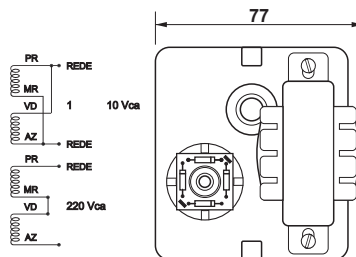
VERSÃO TR COM TRAFO
